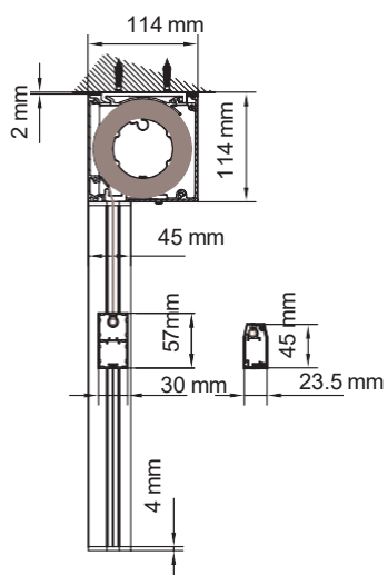
Instalación a techo
