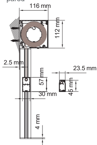
Instalación a pared
